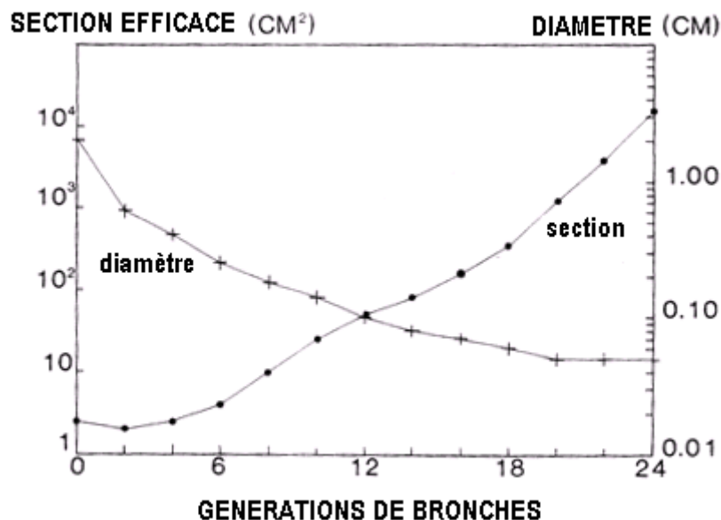
Figure 4 : Diamètre des voies respiratoires et section efficace totale en fonction des générations de bronches, d'après Robinson (110).
